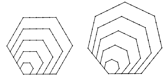
Sechseckszahlen 1, 1+5=6, 1+5+9=15, ... Siebeneckszahlen 1, 1+6=7, 1+6+11=18, ...
